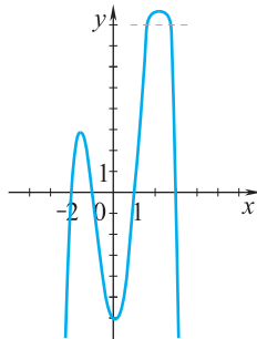
d) x_1 = 1 , x_2 = -1 , x_3 = 3 , x_4 = -2 , p(0) = -6 ,
