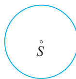
krožnica
