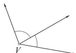
sosednja kota
