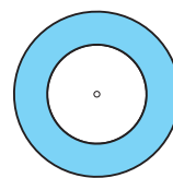
krožni kolobar
