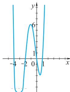
č) x_1 = 1 , x_2 = -2 , x_3 = -4 , x_4 = 0 , p(0) = 0 ,
