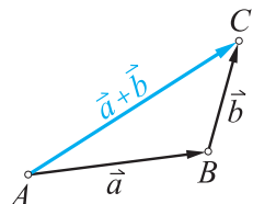
Trikotniško pravilo
