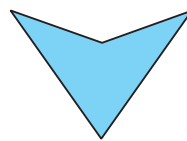
štirikotnik
